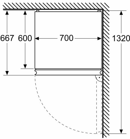
Dimensiones en mm
