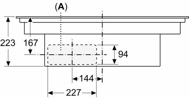
Dimensiones en mm Vista frontal
