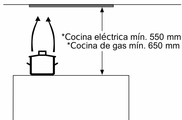
*Cocina eléctrica mín. 550 mm *Cocina de gas mín. 650 mm *desde el borde superior de la parrilla
