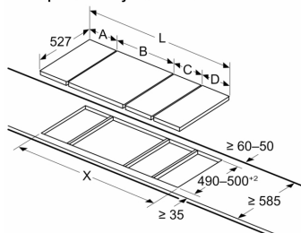
Dimensiones en mm Imagen de la tabla de combinaciones posibles de Domino con los dispositivos correspondientes y las dimensiones del hueco
